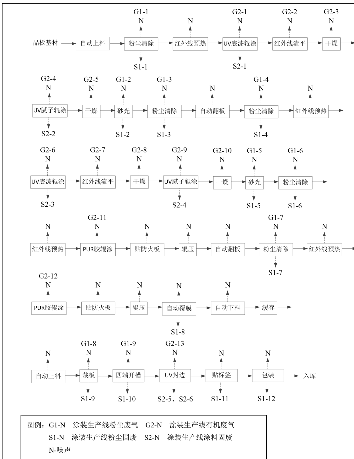
图 5-2 涂装无机复合矿物板工艺流程及产污节点图
