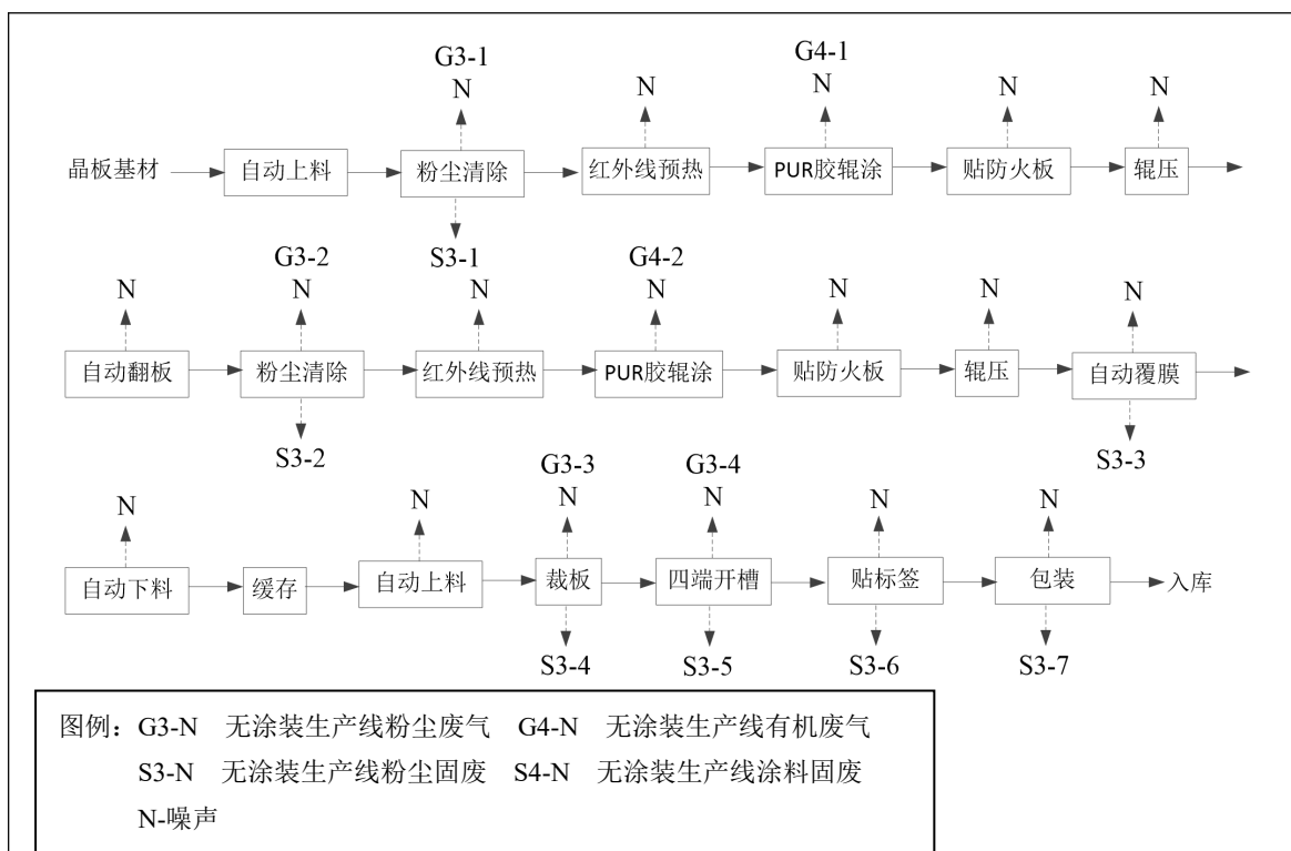
图 5-3 无涂装无机复合矿物板工艺流程及产污节点图
