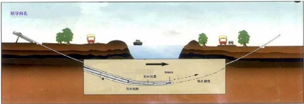
图 2-7-1 钻导向孔示意图
