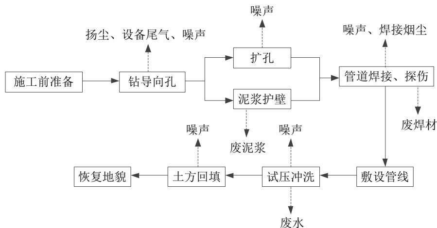
图 2-6 定向钻段施工流程图
