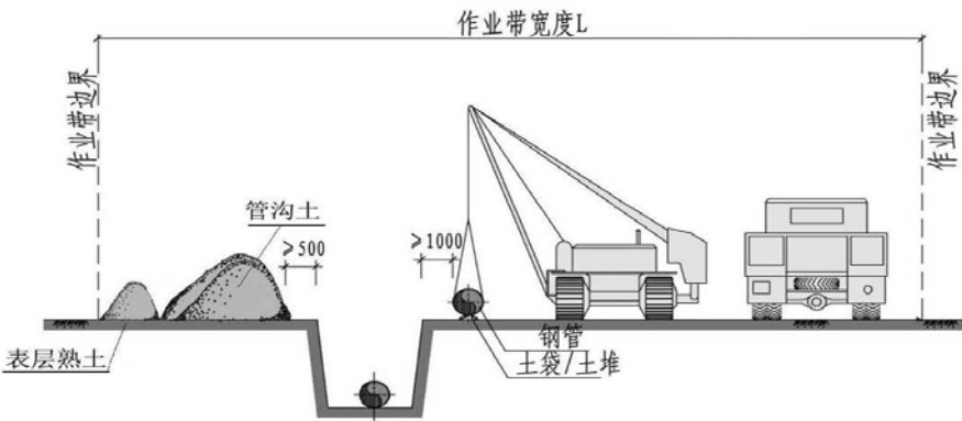
图 2-3 开挖施工工艺作业示意图
