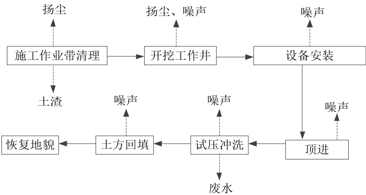
图 2-4 顶管穿越段施工流程图
