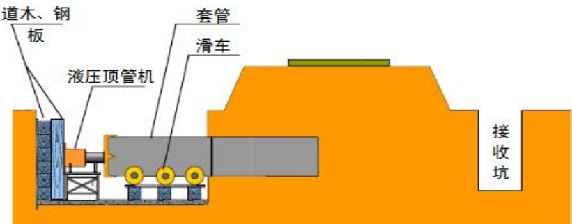
图 2-5 顶管施工工艺作业示意图
