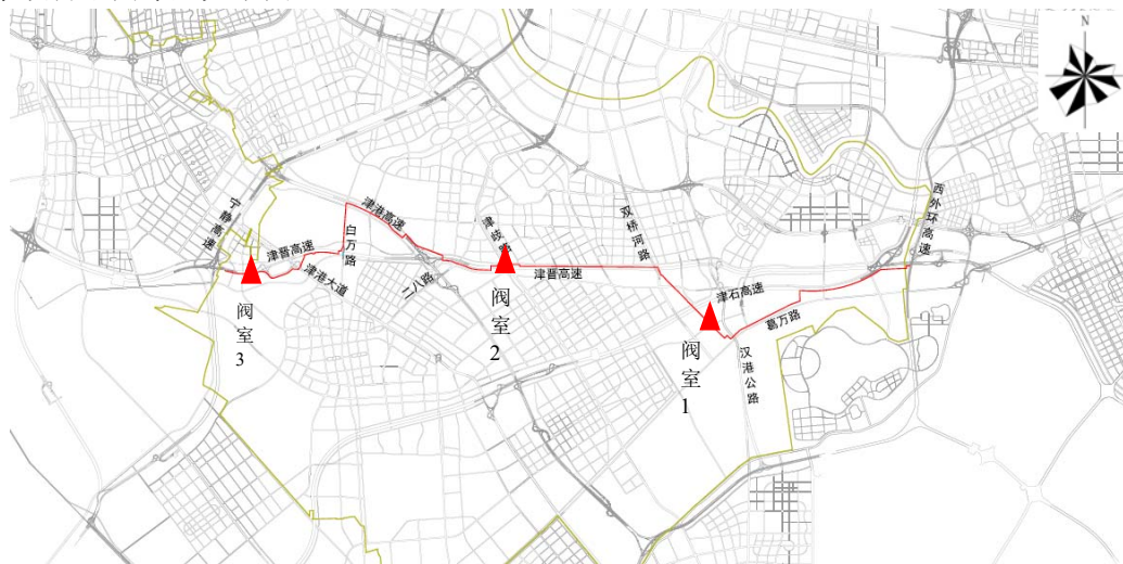
图 2-1 本项目管路走向图
